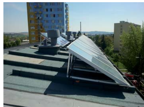
Solární systém na bytovém domě Milevsko
