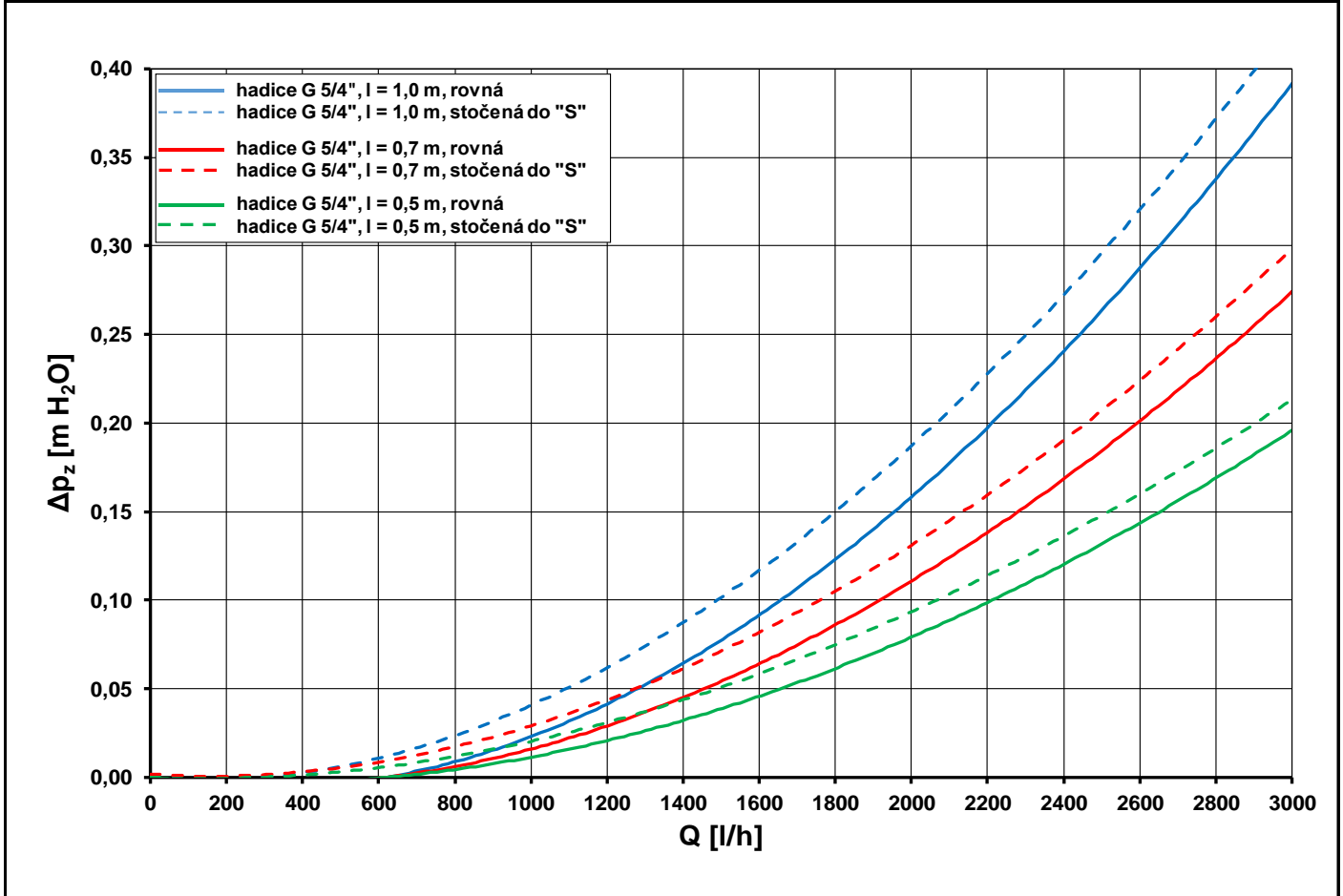
Graf tlakové ztráty pro hadici s přípojením G 5/4"
