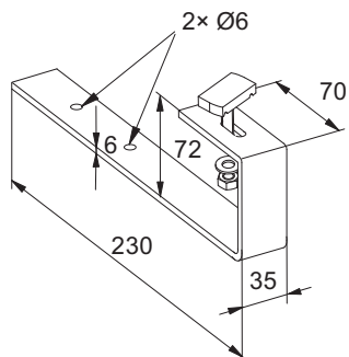
Obr. 9: Hák pro střechy s krytinou z břidlice, šindele nebo plechu
