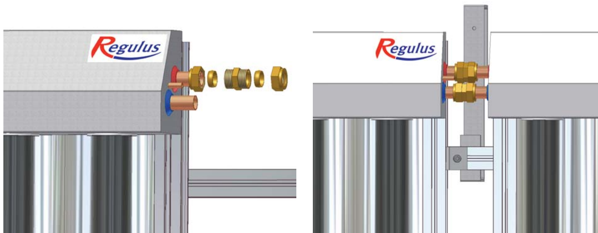
Obr. 24: Spojování kolektorů
