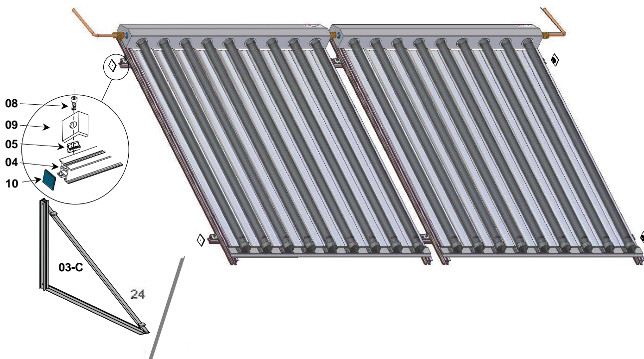
Obr. 15: Trojúhelníková podpěra a zavětrovací vzpěra
