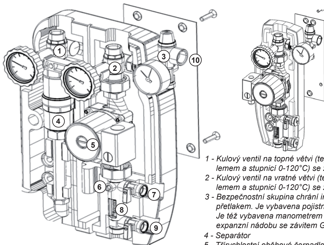
Obr. 29: Čerpadlová skupina
