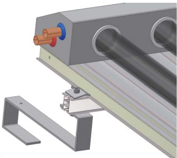
Obr. 14: Montáž upevňovací destičky
