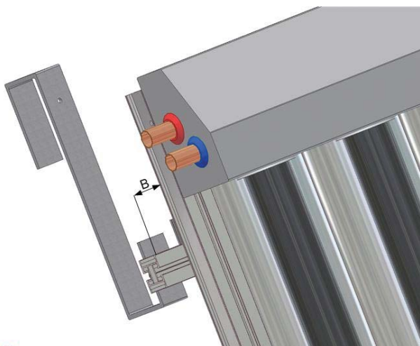
Obr. 13: Vzdálenosti hrany kolektoru a okraje H profilu
