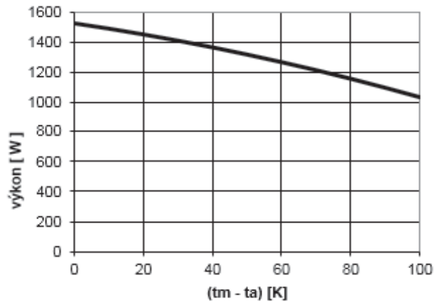
Graf okamžitého výkonu kolektoru při osvětlení 1000 W/m 2
