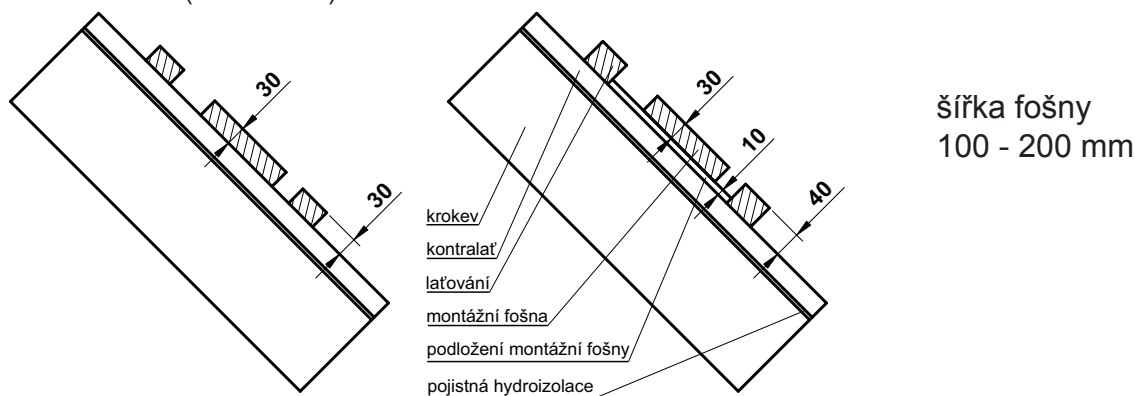
Obr. 2: Dorovnání tloušťky montážní fošny
