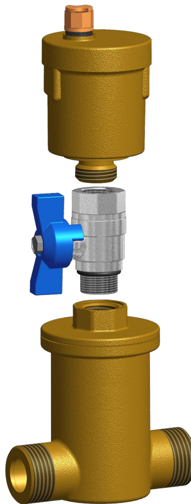
Obr. 30: Vodorovný separátor vzduchu a automatický odvzdušňovací ventil
