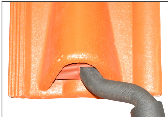
Obr. 14: Průchod potrubí odvětrávací taškou
